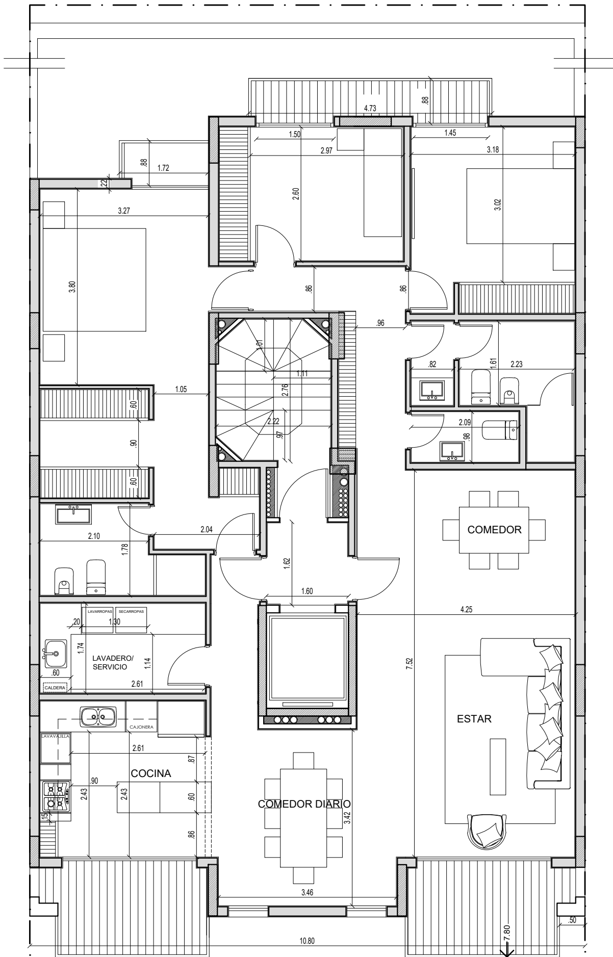
PLANTA PISO LIBERTAD
